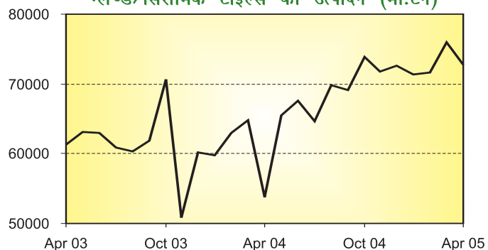
Production of Glazed/ceramic tiles (tonnes) ग्लेज़्ड/सिरामिक टाइल्स का उत्पादन (मी.टन)
